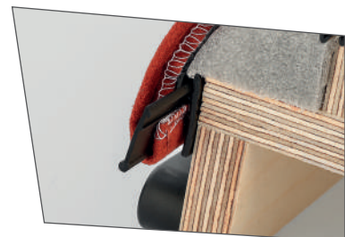
24 | Lock profile with counter-bar Verschlussprofil mit Gegenleiste
